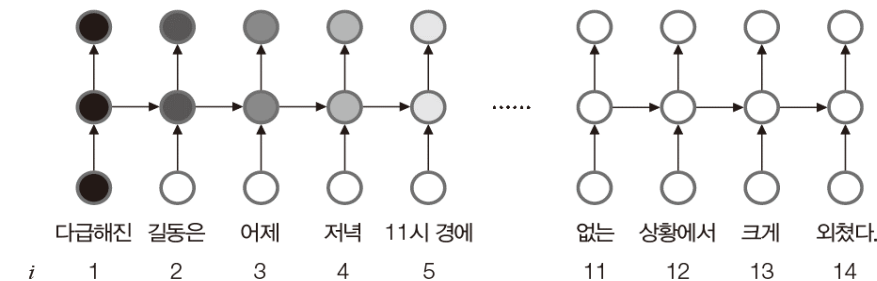
(a) 선별 기억 능력이 없는 순환 신경망
