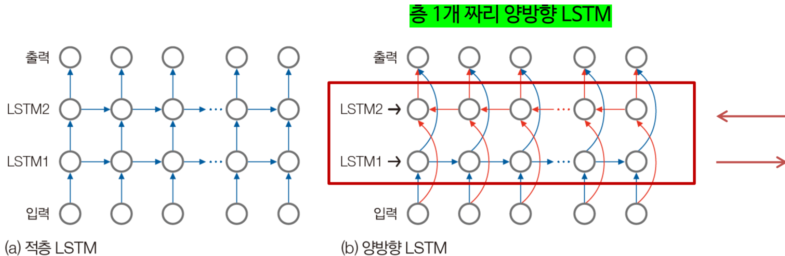
그림 8-8 적층 LSTM과 양방향 LSTM
