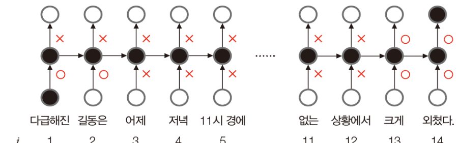
(b) 선별 기억 능력을 지닌 LSTM
